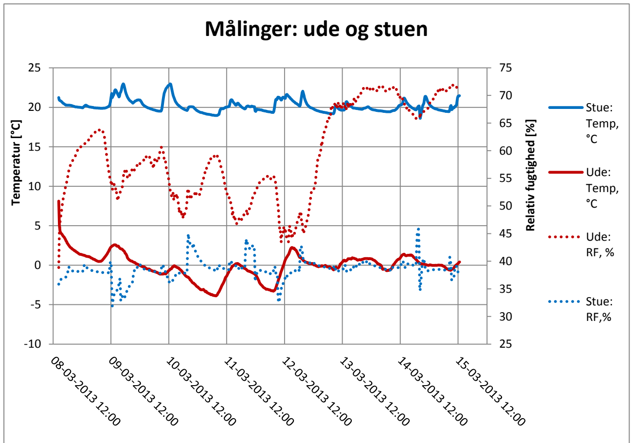
Figur M7- Målinger af relativ fugtighed % og temperatur, stuen og udenfor.
