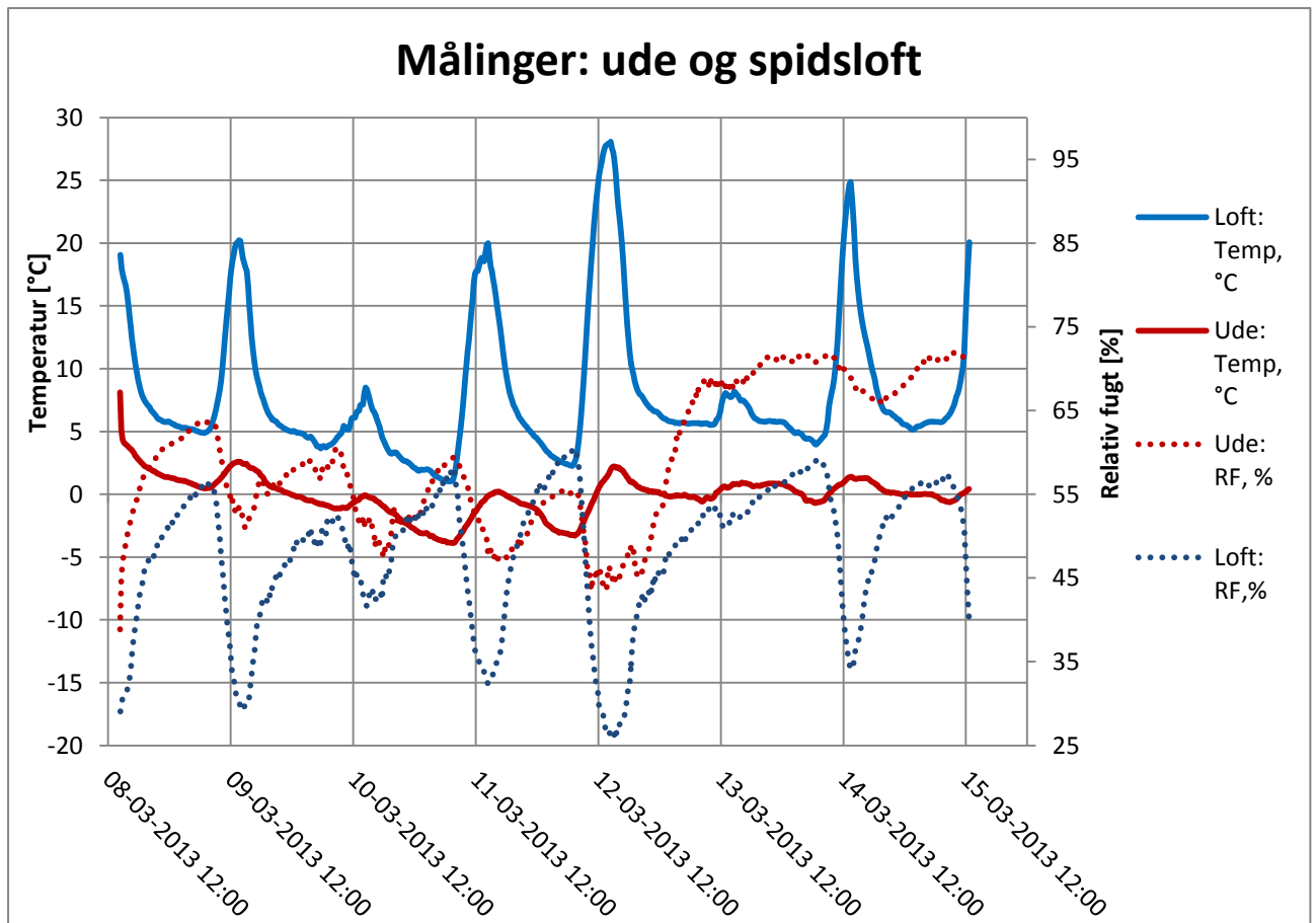
Figur M3 – Målinger af relativ fugtighed % og temperatur, spidsloft og udenfor
