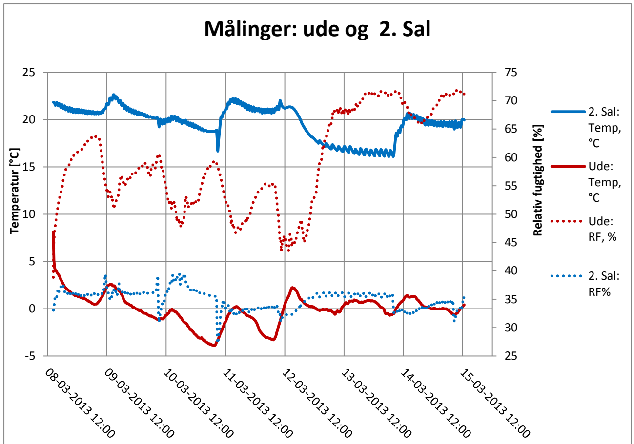
Figur M5 - Målinger af relativ fugtighed % og temperatur, 2.sal og udenfor.
