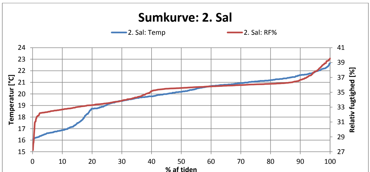
Figur M6 - Sumkurve over målinger af 2 sal, temperatur og relativ fugtighed %.
