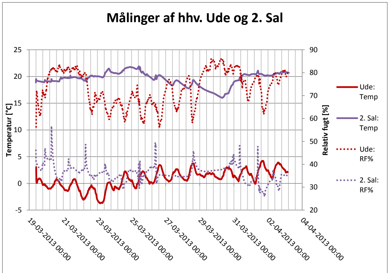
Figur N 5 - Målinger af relativ fugtighed % og temperatur, 2. sal og udenfor.
