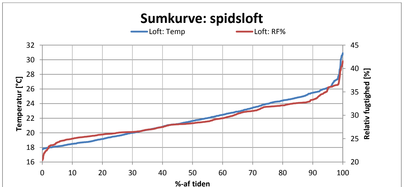
Figur N 4 - Sumkurv over temperatur og relativ fugtighed % for spidsloft.
