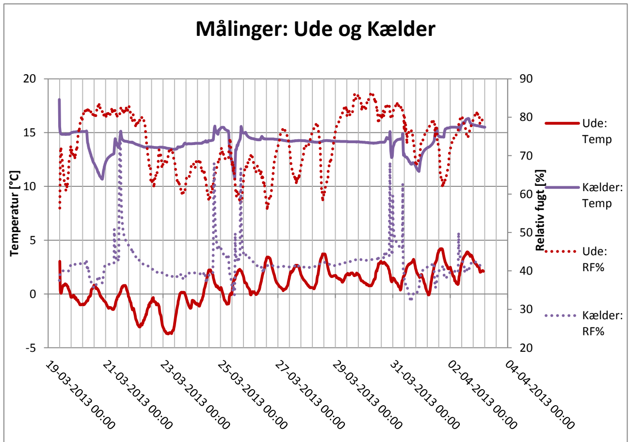
Figur N 1- Målinger af relativ fugtighed % og temperatur, kælder og udenfor.
