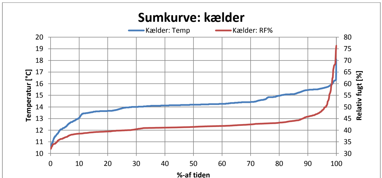
Figur N 2 – Sumkurve over målinger af kælder, temperatur og relativ fugtighed %
