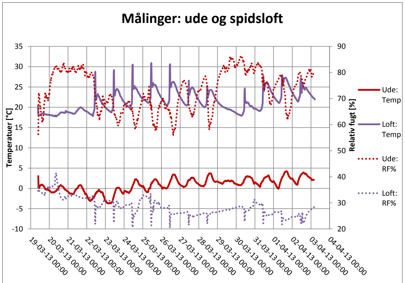
Figur N 3 - Målinger af relativ fugtighed % og temperatur, spidsloft og udenfor.
