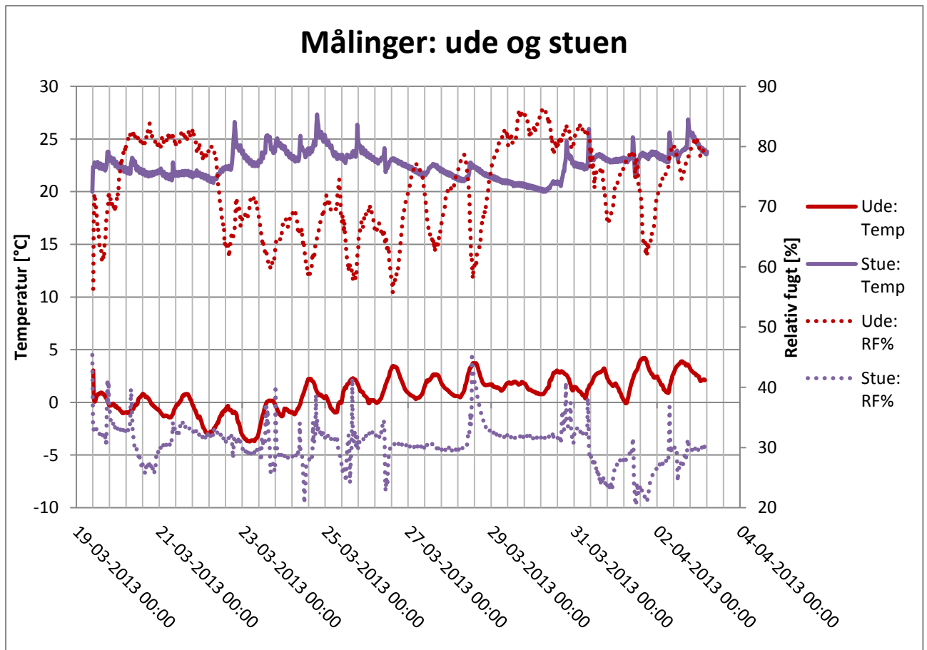
Figur N 7 - Målinger af relativ fugtighed % og temperatur, stuen og udenfor.
