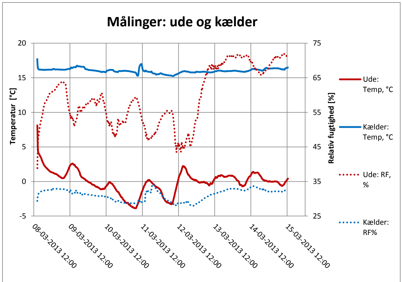
Figur M1 - Målinger af relativ fugtighed % og temperatur, kælder og udenfor.
