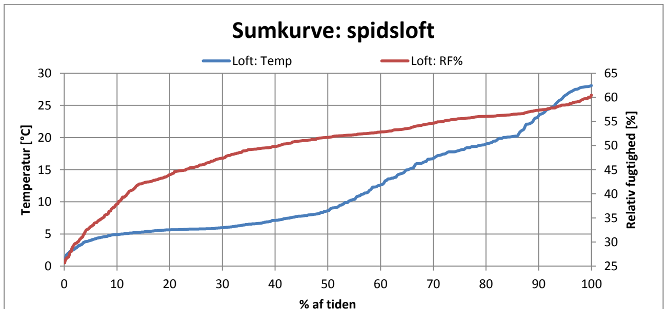
Figur M4 - Sumkurve over målinger af spidsloft, temperatur og relativ fugtighed %
