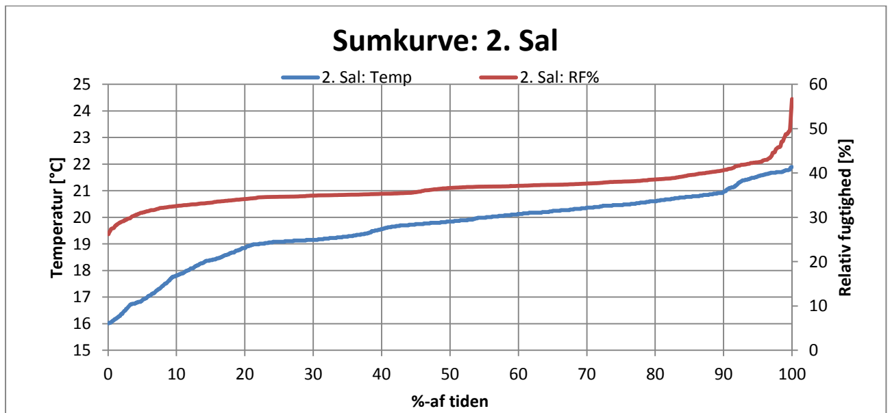
Figur N 3 - Sumkurve over måling af 2 sal, temperatur og relativ fugtighed %.
