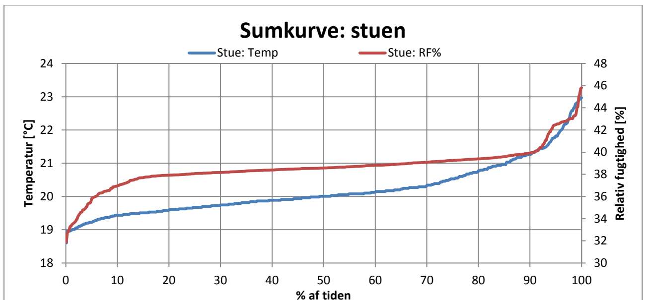
Figur M8 - Sumkurve over målinger af stuen, temperatur og relativ fugtighed %.
