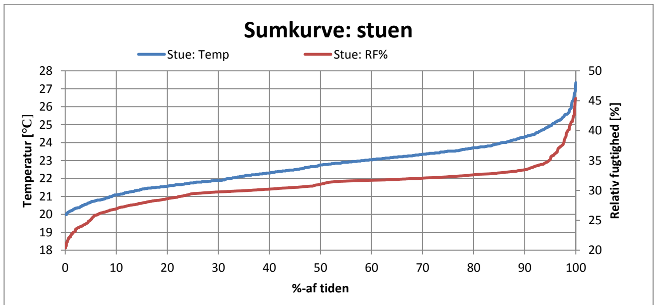
Figur N 8 - Sumkurve over målinger af stuen, temperatur og relativ fugtighed %.
