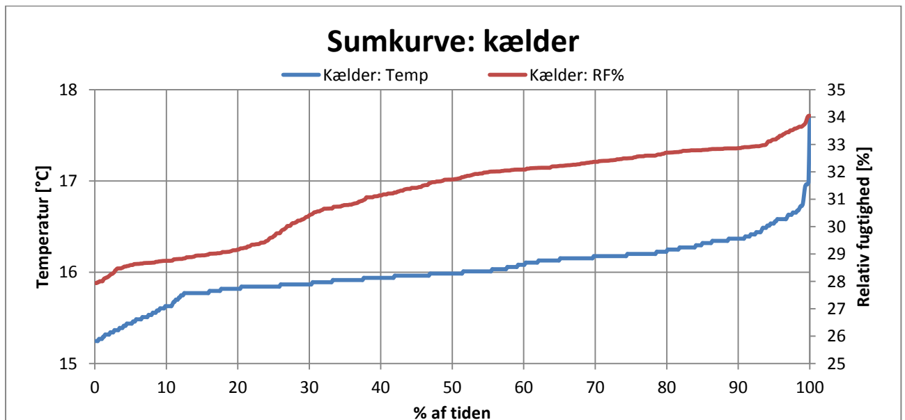
Figur M2 – Sumkurve over målingerne af kælder, temperatur og relativ fugtighed %.
